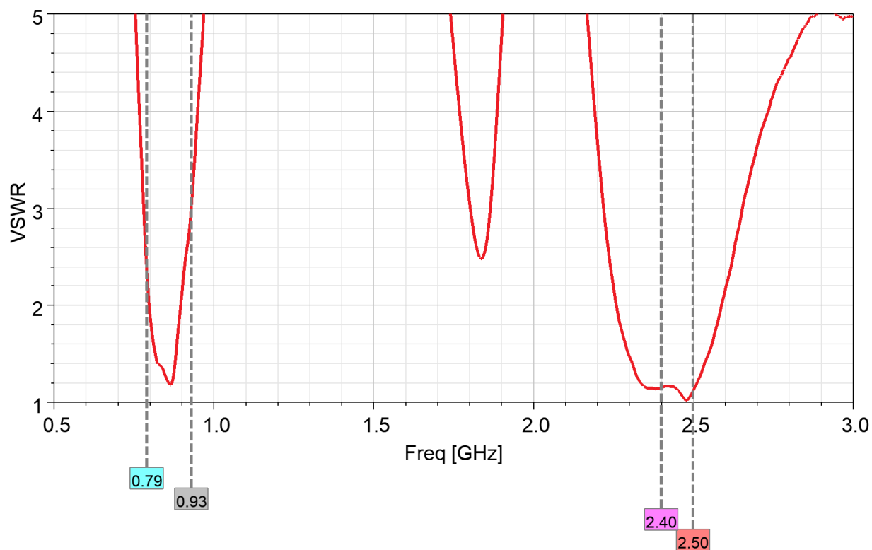
VSWR
