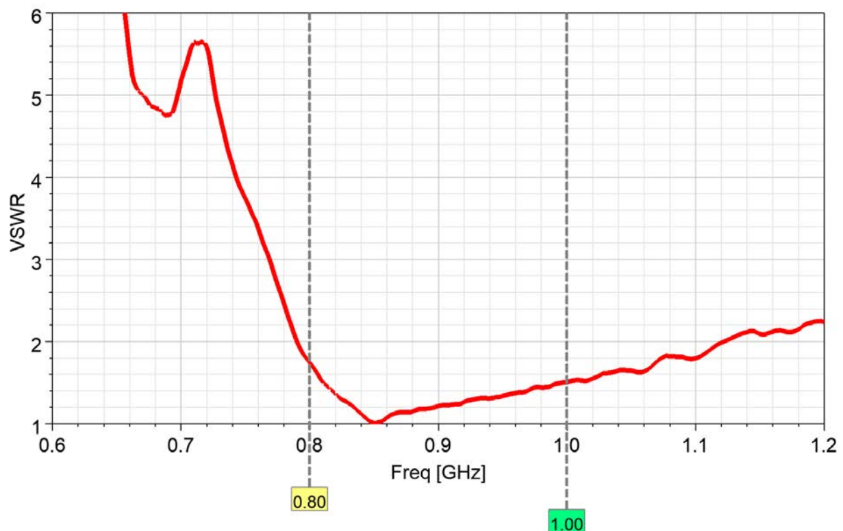
VSWR
