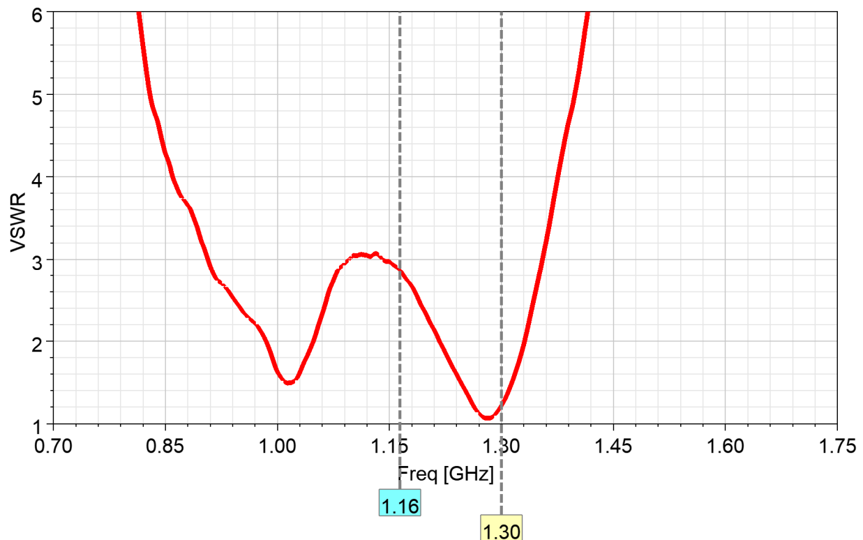
VSWR
