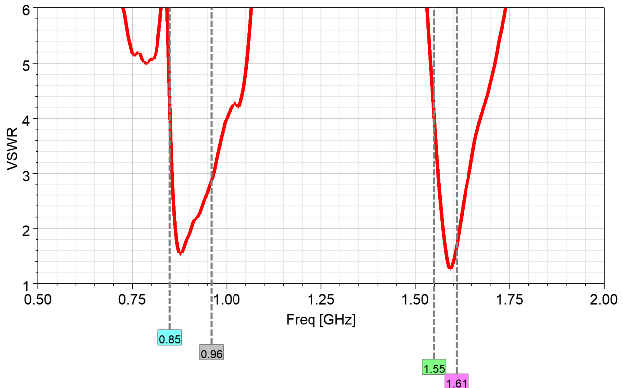
VSWR
