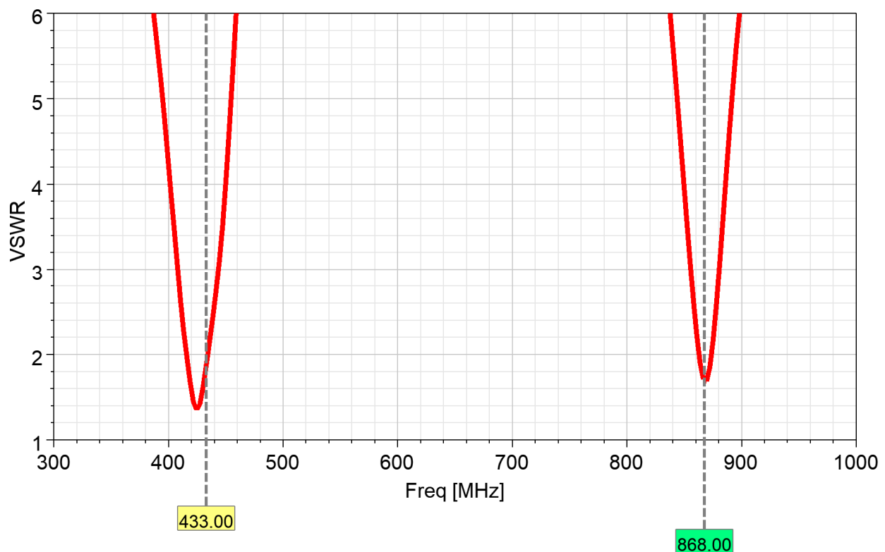
VSWR
